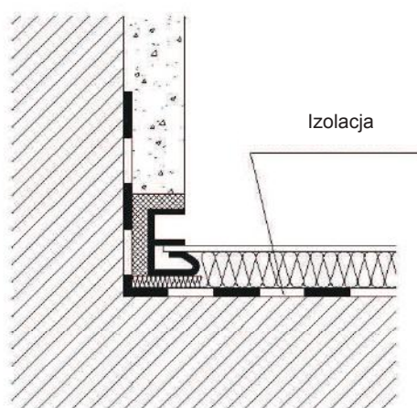
Otwarte części czołowe nowe budownictwo
