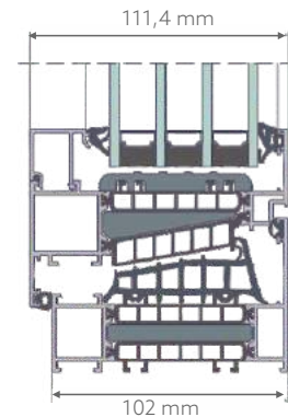
PRZEKRÓJ PRZEZ OKNO TM 102HI
