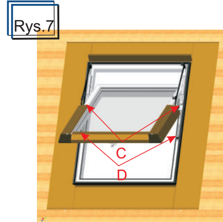
W odwrotnej kolejności jak na rys. 3 włożyć skrzydło w ościeżnicę tak by rolki ślizgowe okucia skrzydłowego C znalazły się w gnieździe listwy ślizgowej D rys. 7. Trzymając skrzydło za ramiona wpiąć okucie ramienia w okucie ościeżnicy jak na rys. 3a. Dokręcić wkręty zaciskowe B rys. 3 momentem 2,5 Nm.
