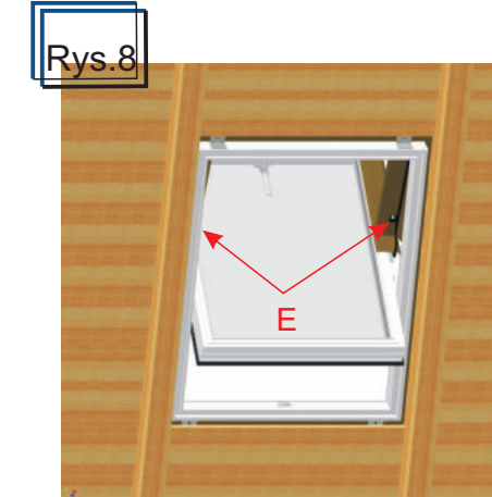
Zamocować zespół górny blach, wpinając go w gniazda ramion nośnych E oraz dokręcając wkręty jak na rys. 2a.
