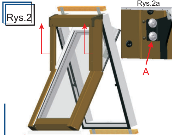
Przed przystąpieniem do montażu, ustawić okno jak na rys. 2 podkładając pod skrzydło miękki materiał np. styropian. Aby wyjąć skrzydło z ościeżnicy zdjąć zespół górny obłachowania, w tym celu: - odkręcić wkręty mocujące A pod obłachowaniem - lekko odchylić i zsunąć obłachowanie do góry (wg strzałek)
