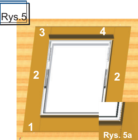
W celu zamontowania kołnierza uszczelniającego należy wyjąć uszczelkę naramową, zamocować kolejno elementy kołnierza jak na rys. 5a.
