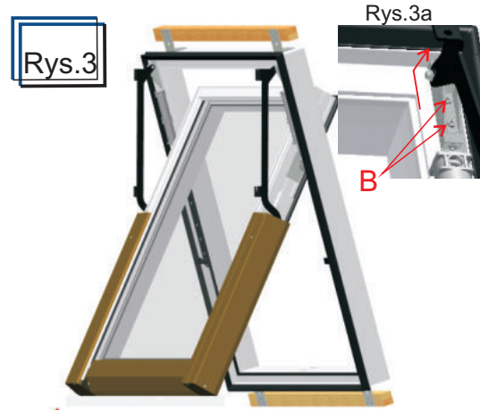
Po zdjęciu zespołu górnego blach poluzować wkręty zaciskowe B i rozpiąć okucie w kierunku pokazanym na rys. 3a. Czynnność wykonać dla lewej i prawej strony. Wyjąć skrzydło ostrożnie odkładając na miękki i czysty materiał np. styropian lub wełnę izolacyjną. Odkręcić dolną i górną listwę transportową.
