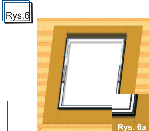
Zamocowany w ościeżnicy kołnierz uszczelniający przykryć uszczelką naramową, wciskając ją w rowek ościeżnicy jak na rys. 6a.
