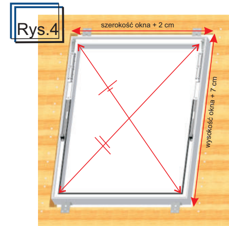
Przygotować otwór pod ościeżnicę w więźbie dachowej jak na rys. 4 do istniejącego deskowania. Przykręcić ościeżnicę, wkręcając po trzy wkręty w każdy kątownik montażowy.
